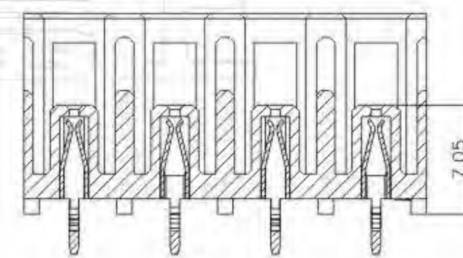
A-A SECTION
