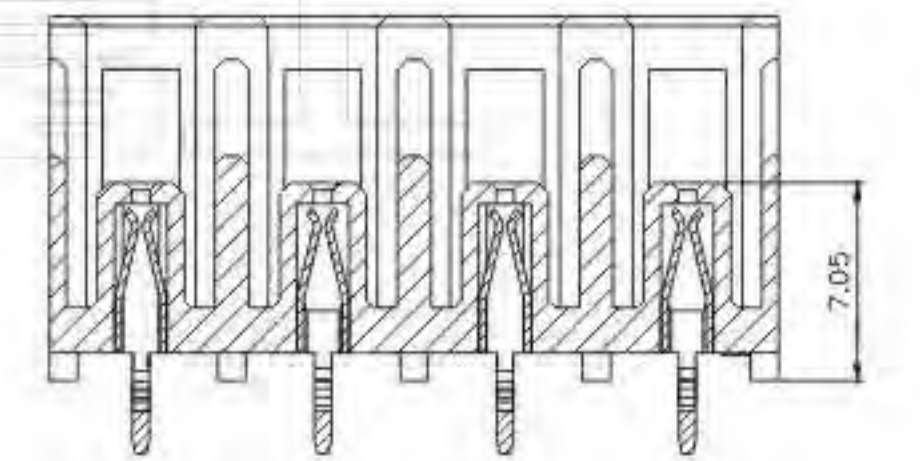
A-A SECTION
